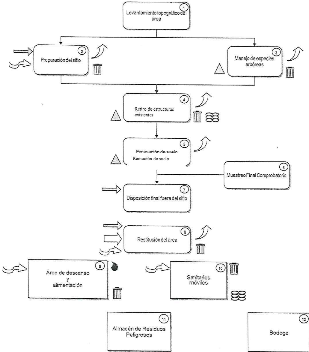
Figura 2. Diagrama del proceso de remediación del área contaminada
