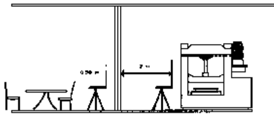
FIGURA N° 25. POSICIÓN DEL MICROFONO DE MEDICIÓN PARA DETERMINAR EL AISLAMIENTO DEL MURDO, BARRA, ETC DEL PROYECTO EDUCATIVO. RUMONOTECOLIBRI
